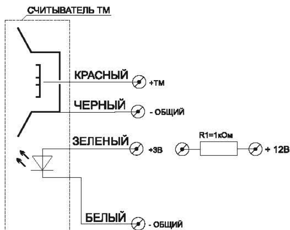
Рис.1 Схема считывателя электрическая, принципиальная
